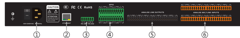
主机后面板示意图
